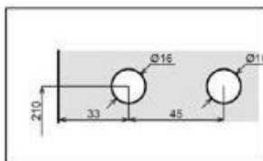
Схема сверления под петли GT
